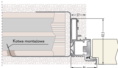
Ościeżnica do ściany murowanej
