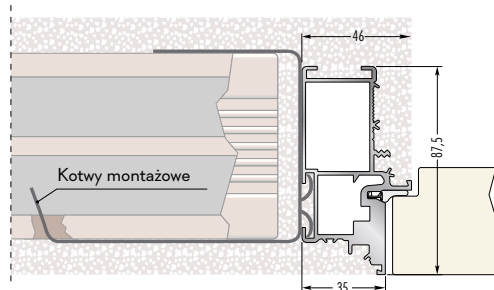
Ościeżnica do ściany murowanej
